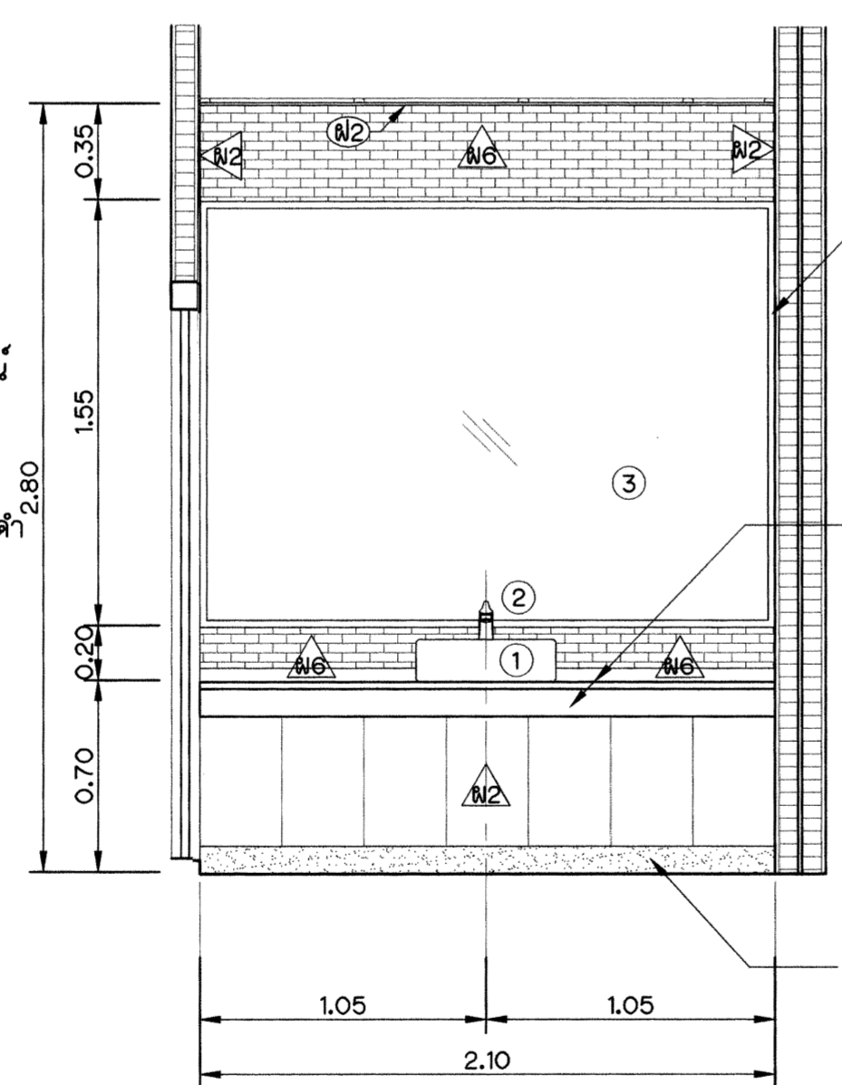
รูปตัด ข - ข มาตราส่วน 1 : 25
