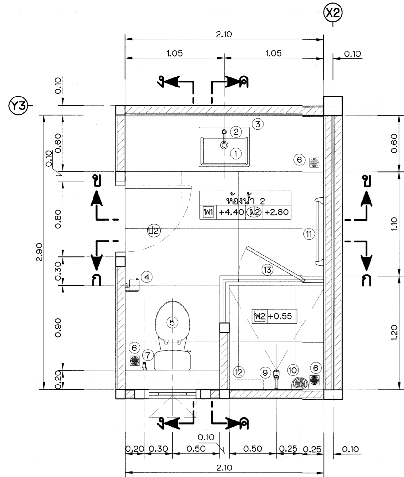
ขยายแปลนขยายห้องน้ำ 1 มาตราส่วน 1 : 25
