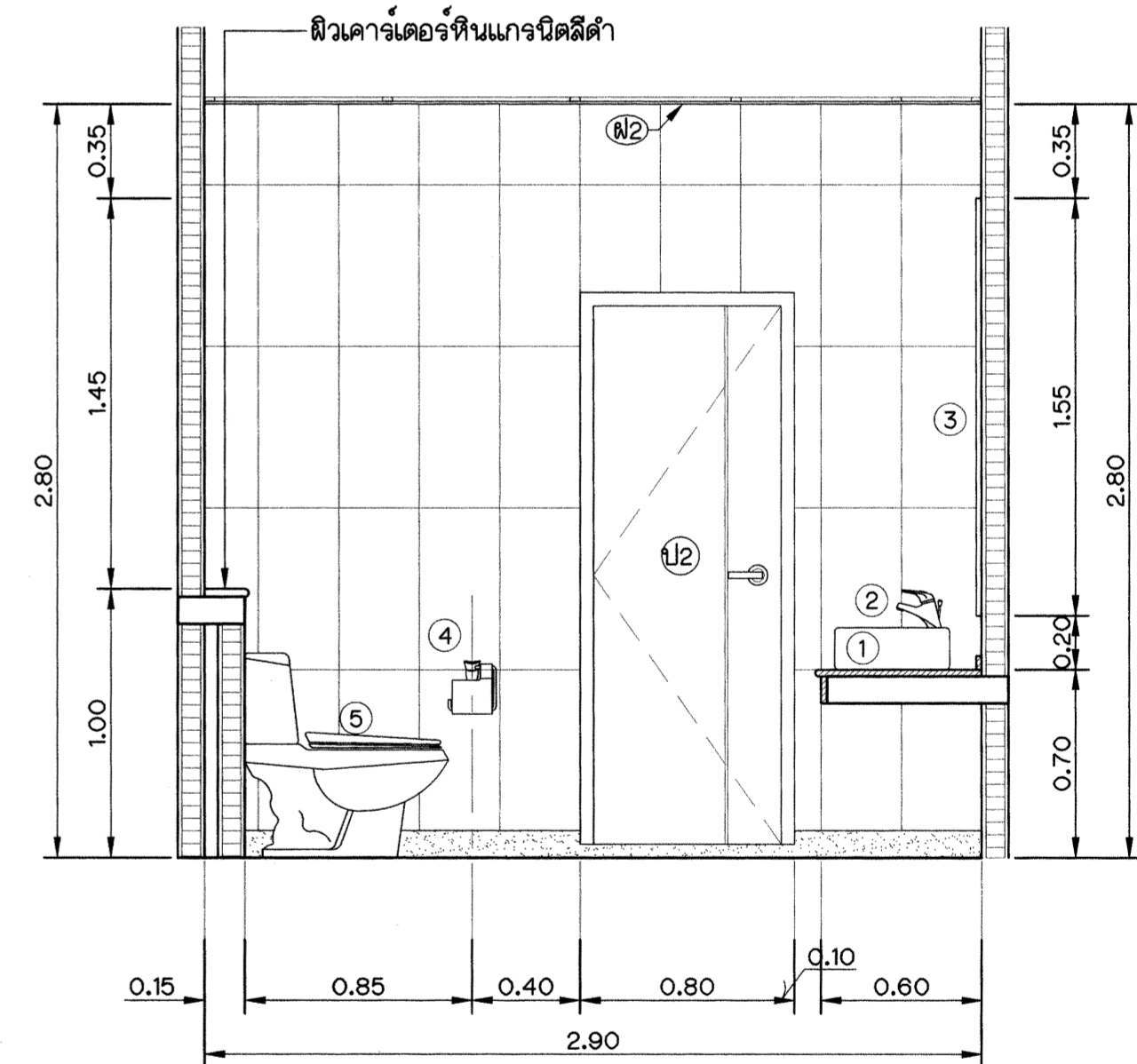
รูปตัด ง - ง มาตราส่วน 1 : 25
