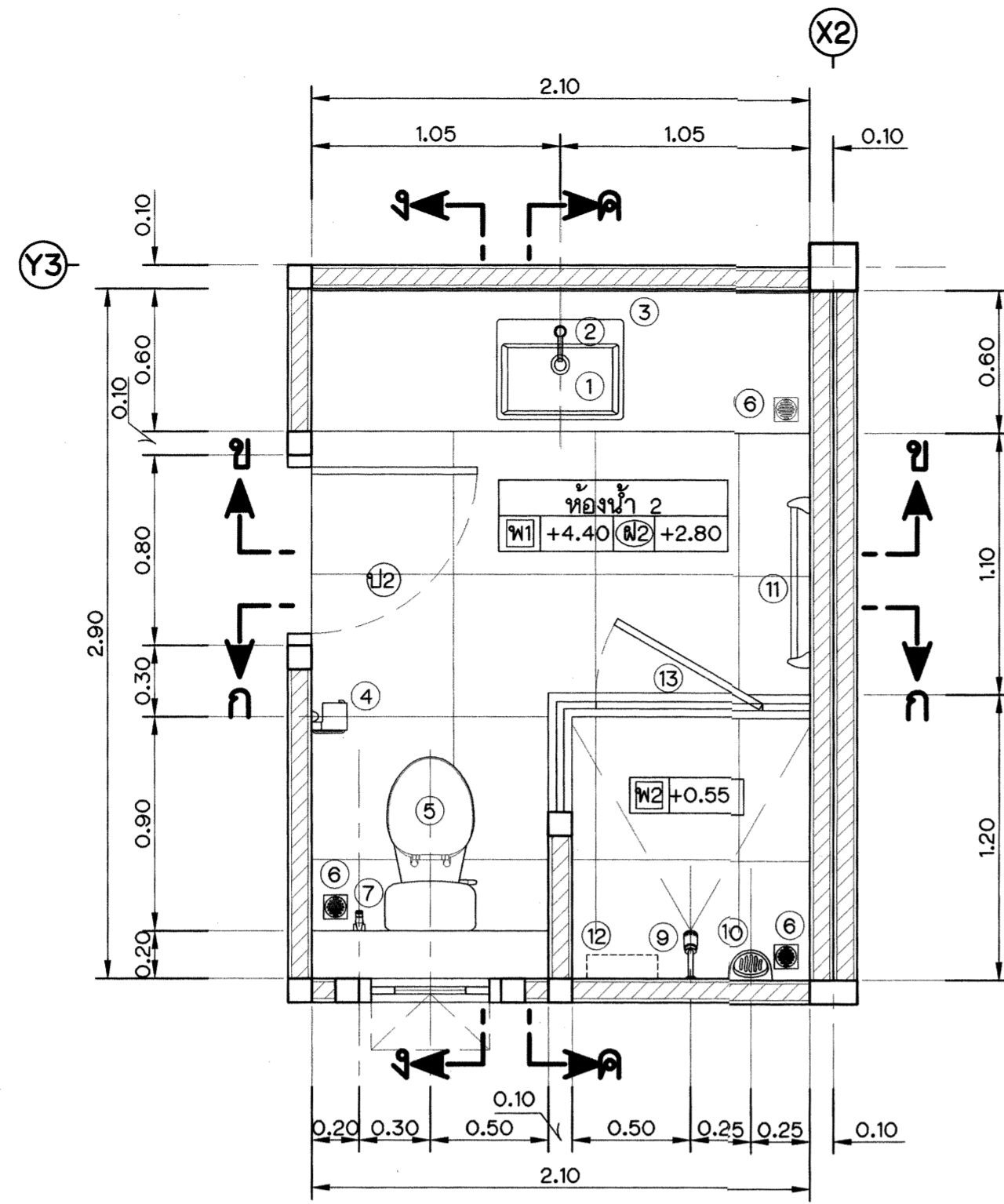
แปลน มาตราส่วน 1 : 25
